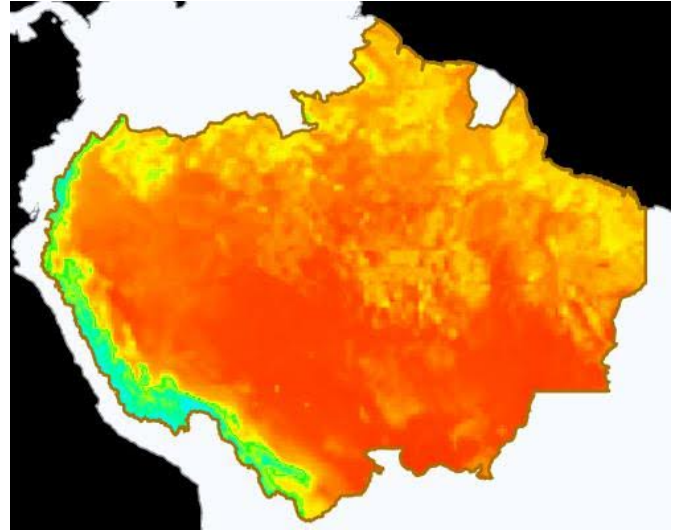
Pronóstico de Temperatura Máxima para el día 13/06/2024
