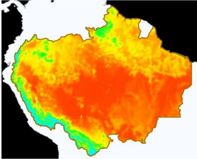
Pronóstico de Temperatura Máxima del día 10/06/2024
