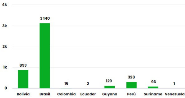
Número de nuevos eventos de Incendios-Quemas activados por País el día 02/10/23
