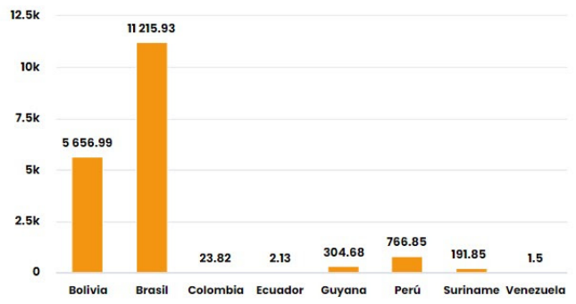
Hectáreas (miles) de área proyectada afectadas por nuevos eventos por País el día 02/10/23
