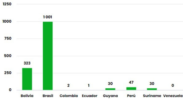
Número de nuevos eventos de Incendios-Quemas activados por País el día 02/10/23
