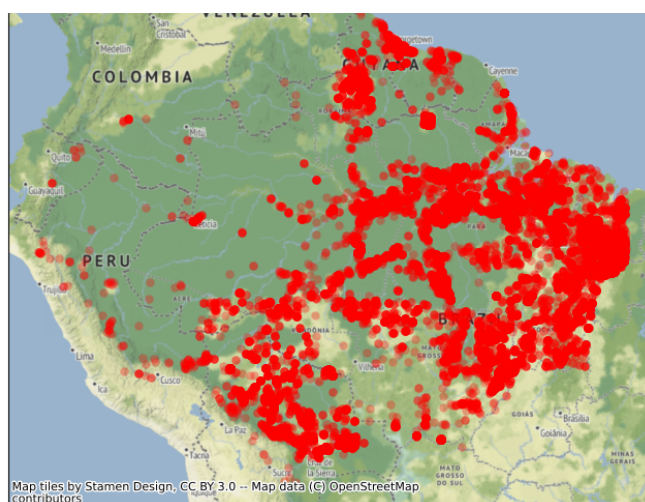
Mapa de Distribución de focos de calor detectados el día 01/10/2023
