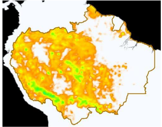
Pronósticos de Precipitación para el día 25/11/2023
