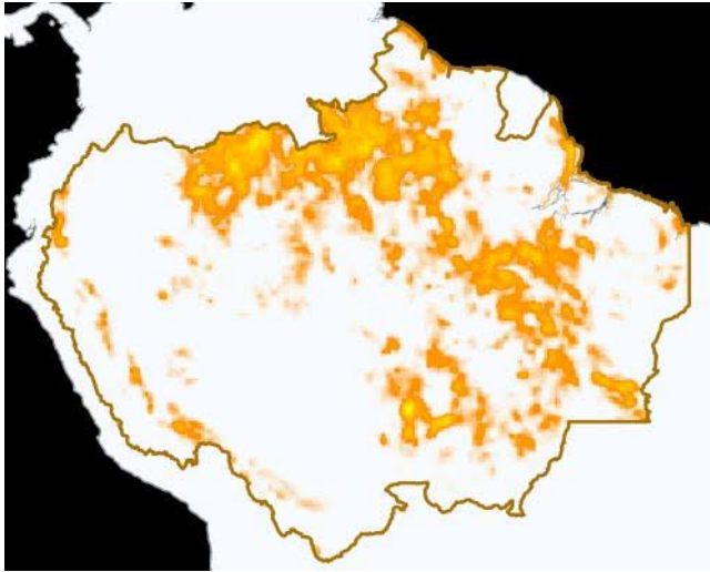
Pronósticos de Precipitación del día 22/11/2023
