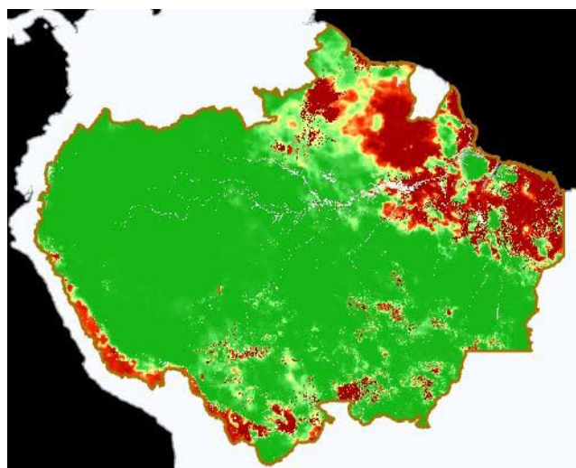
Pronóstico de Riesgo de Fuego para el día 25/11/2023
